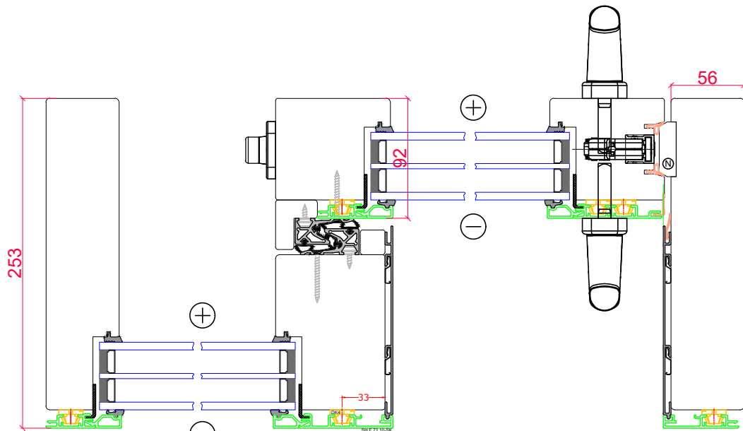
horisontaalne lõige avatav-kinnine osa
