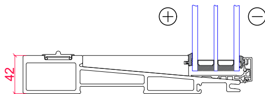
vertikaalne lõige kinnine osa
