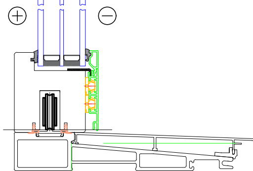
vertikaalne lõige avatav osa
